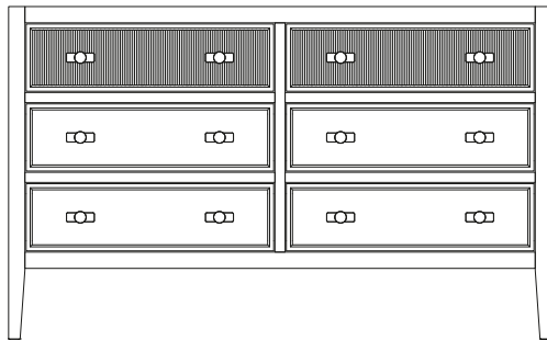
3 + 3 WIDE CHEST H: 818 W: 1330 D: 450
