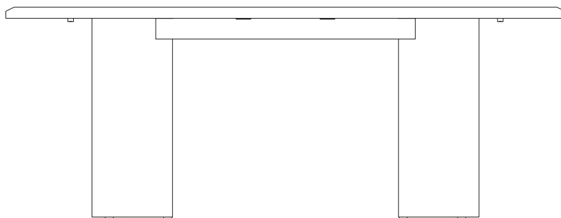
DINING TABLE H: 750 W: 2000 D: 1000
