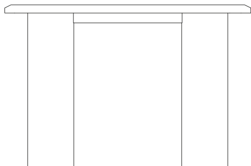
CONSOLE TABLE H: 790 W: 1200 D: 400
