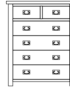
4+2 CHEST H: 1179 W: 970 D: 425
