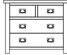
2+2 CHEST H: 773 W: 970 D: 425
