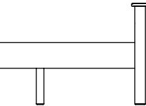
3' LOW FOOT END BED H: 1045 W: 1048 D: 2080
