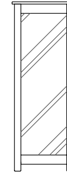
CHEVAL MIRROR H: 1470 W: 550 D: 75
