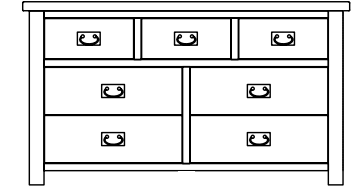
3 OVER 4 CHEST H: 773 W: 1380 D: 425
