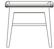
DRESSING TABLE STOOL H: 500 W: 500 D: 350
