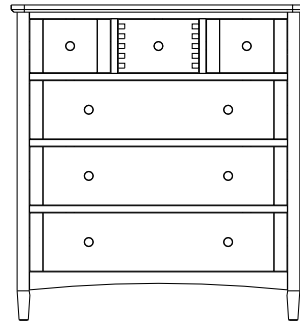
3 + 3 CHEST H: 965 W: 900 D: 450
