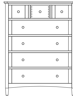
3 + 4 CHEST H: 1165 W: 900 D: 450
